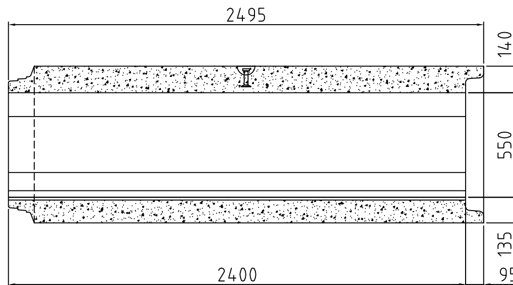
Longitudinal section
